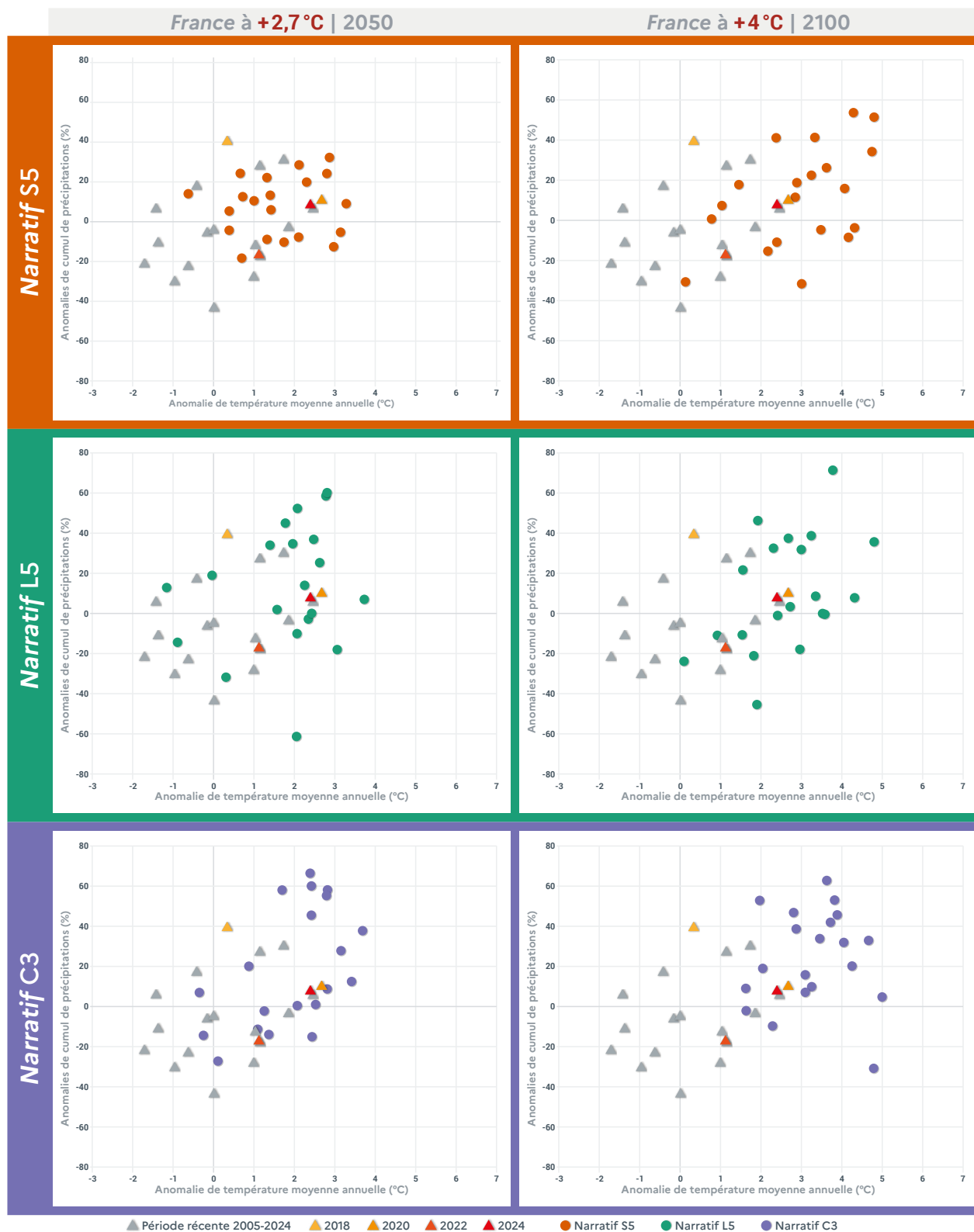
Figure 7 : Évolution de la variabilité interannuelle des narratifs S5, L5, C3, pour l'écart à la moyenne hivernale de température et l'écart relatif du cumulé hivernal de précipitation (référence 1976–2005) selon la période récente 2005-2024 sous forme de triangle gris. Les années 2024, 2022, 2020 et 2018 sont représentées respectivement en rouge, orange foncé, orange et jaune. Les niveaux de réchauffement +2,7°C et +4°C France hexagonale sous forme de ronds de la couleur de la famille concernée en 2050 et 2100.
